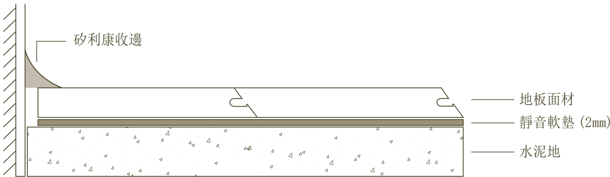
直鋪式
